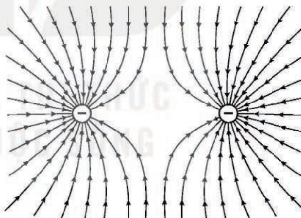
Hình 17.7. Điện phổ của hai điện tích âm Q_1 = Q_2 < 0 đặt gần nhau
