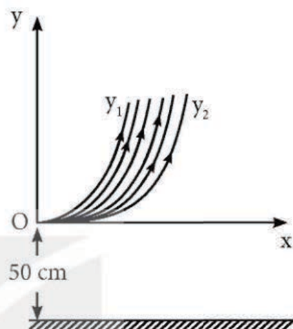
Hình 18.2. Quỹ đạo chuyển động của chùm ion âm
