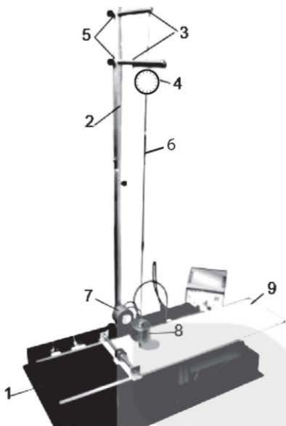
a) Bộ thí nghiệm khảo sát dao động tắt dần của con lắc đơn
