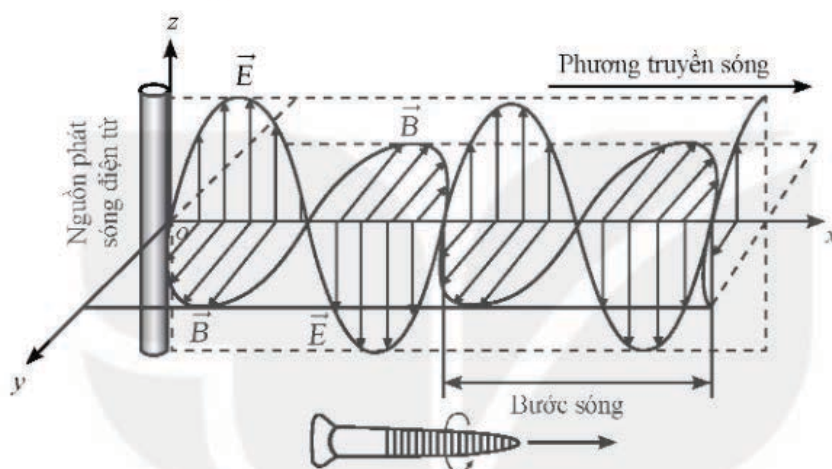
Hình 11.1. Sự lan truyền của sóng điện từ
