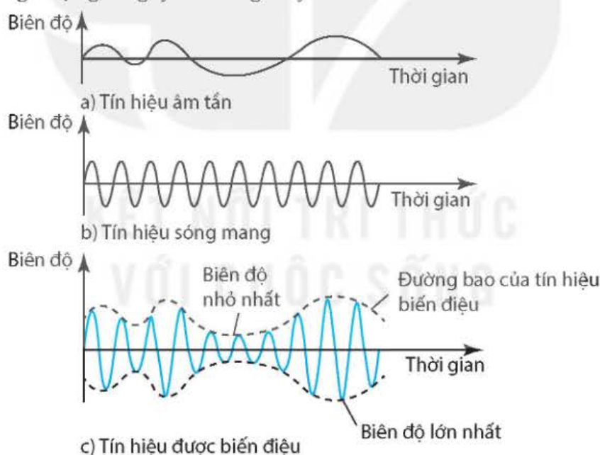
Hình 4.1. Biến điệu biên độ
