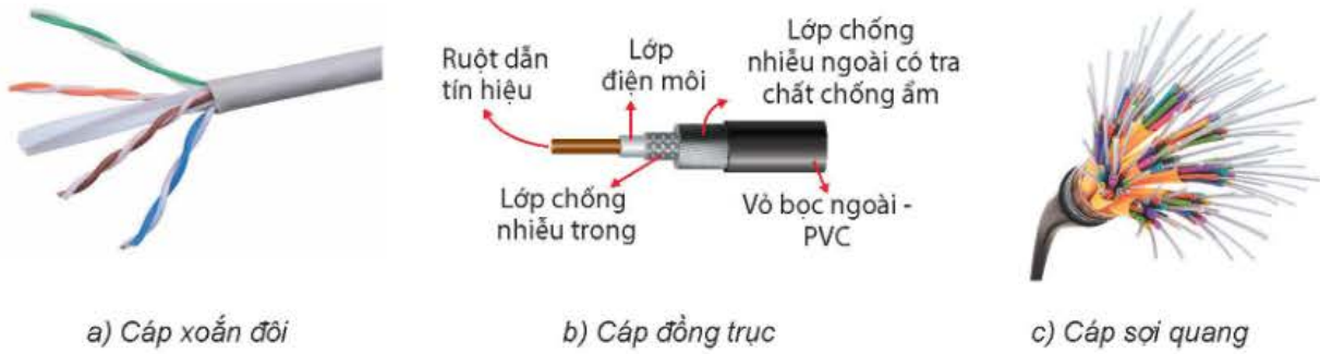
Hình 6.3. Các loại cáp truyền dẫn
