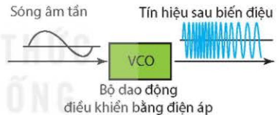
Hình 4.6. Sơ đồ nguyên lý biến điệu tần số
