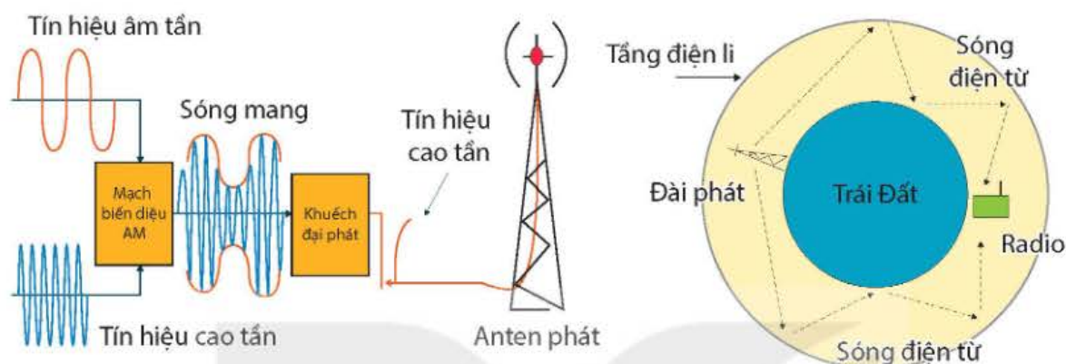
Hình 4.9. Quá trình phát sóng radio AM và việc thu tín hiệu khi đài phát ở xa máy thu
