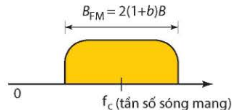
Hình 4.7. Bảng thông của tín hiệu FM
