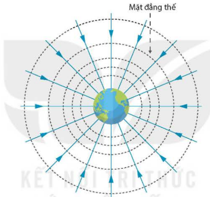
Hình 3.3. Mặt đẳng thế
