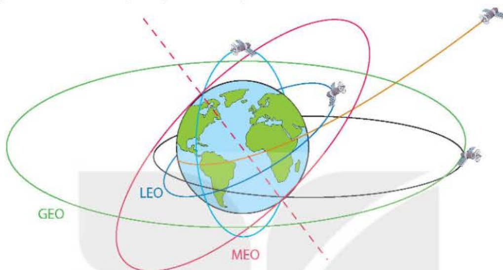
Hình 3.4. Mô phỏng một số quỹ đạo của vệ tinh Trái Đất
