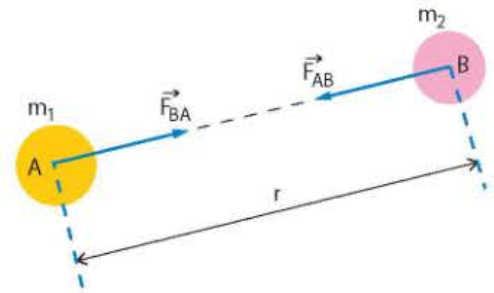
Hình 1.3. Biểu diễn lực hấp dẫn tương tác giữa hai vật A và B.
