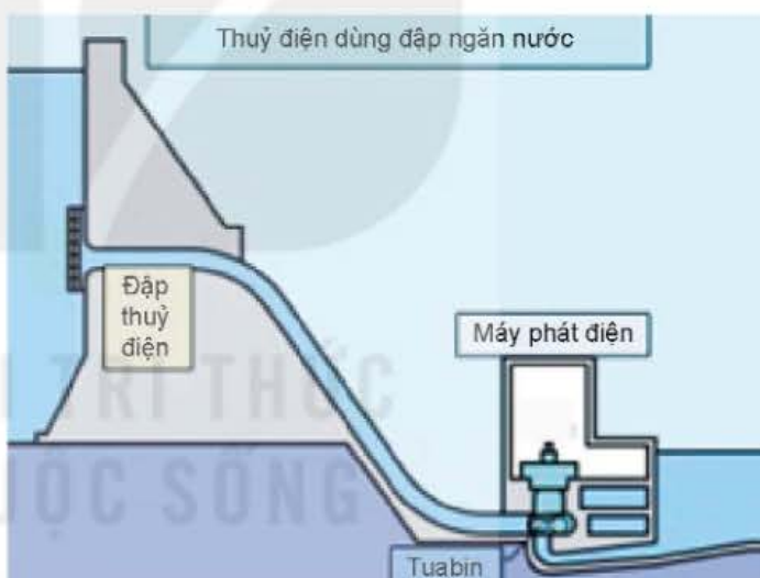
Hình 10.2. Nguyên lí hoạt động nhà máy thủy điện
