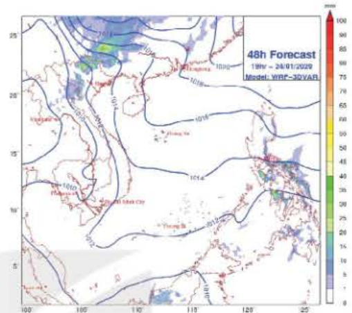
Hình 3.16. Bản đồ thời tiết của Việt Nam, ngày 24 tháng 1 năm 2020
