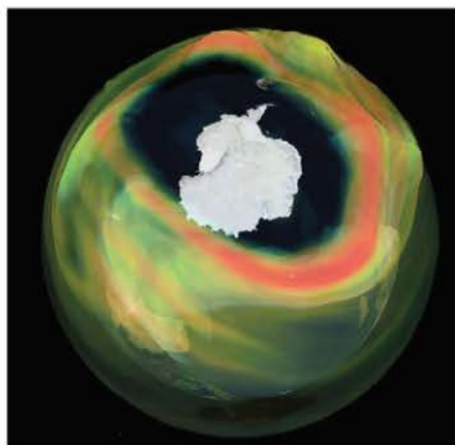
Hình 9.6. Lỗ thủng tầng ozone ở Nam Cực
