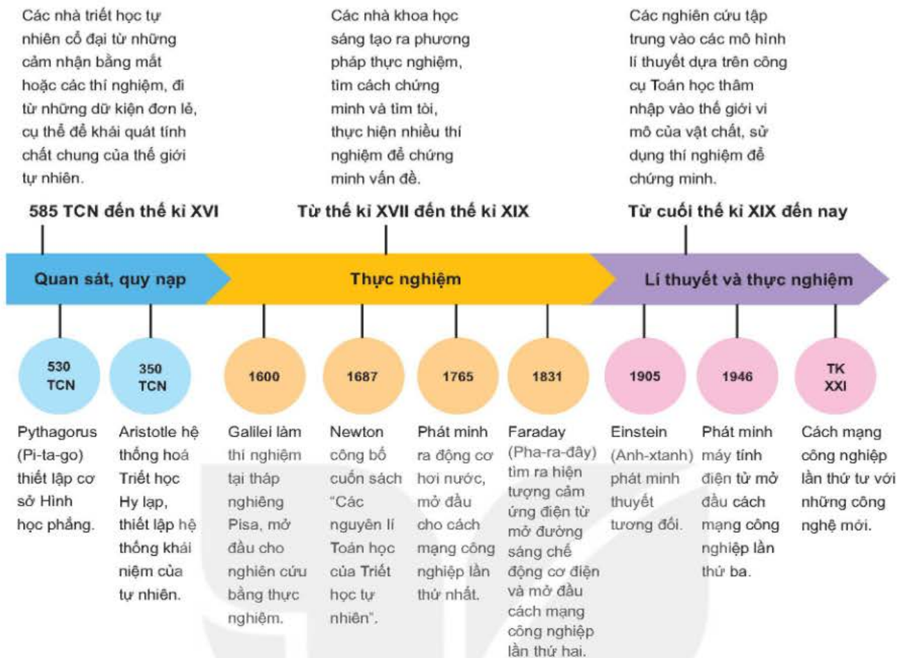
Hình 1.2. Quá trình phát triển của Vật lí học
