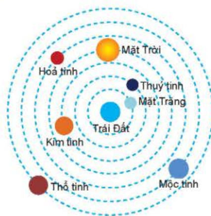
Hình 5.13. Mô hình hệ địa tâm của Ptolemy
