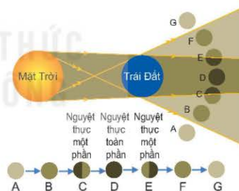
Hình 6.9. Các pha nguyệt thực
