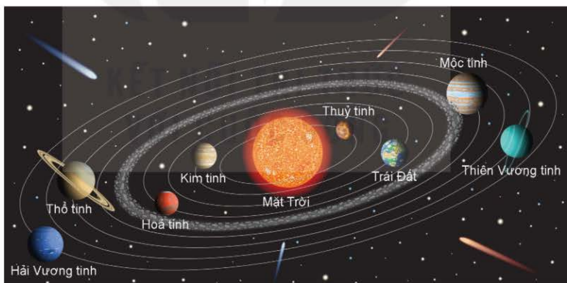
Hình 5.1. Mô hình hệ Mặt Trời
