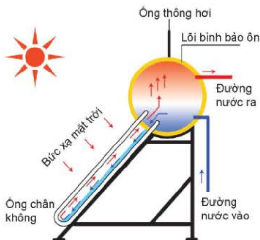
Hình 10.5. Sơ đồ nguyên lí máy nước nóng năng lượng mặt trời
