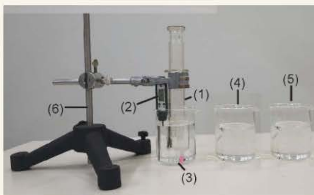
Hình 10.3. Bộ thí nghiệm minh họa định luật Charles
