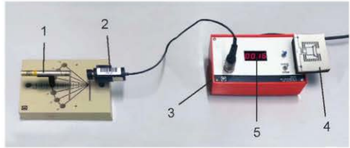
Hình 23.2. Thí nghiệm đếm tia phóng xạ
