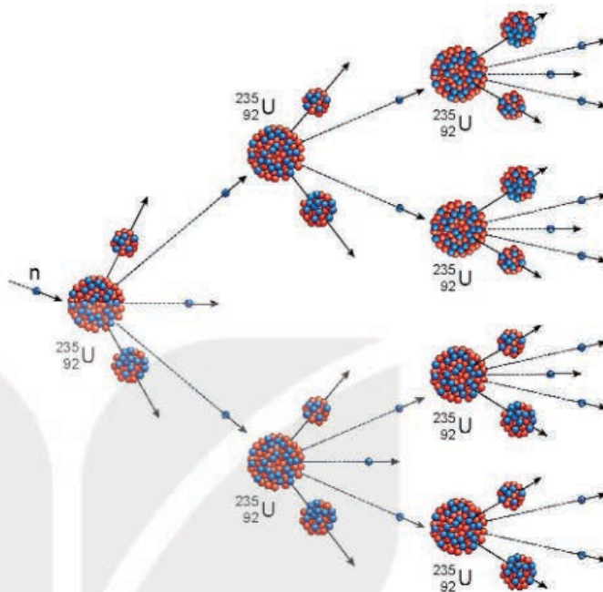
Hình 22.7. Minh họa phản ứng phân hạch dây chuyền với k > 1
