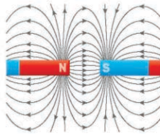
a) Đường sức từ của nam châm thẳng
