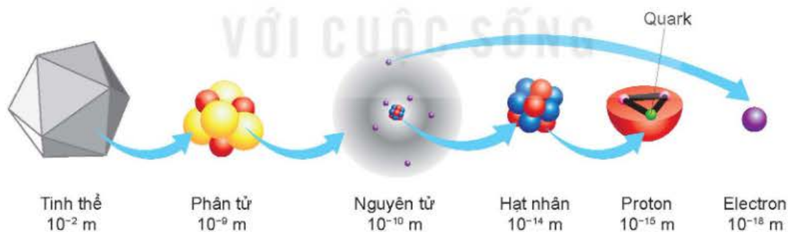
Hình 21.7. Cỡ kích thước của một số loại hạt vi mô
