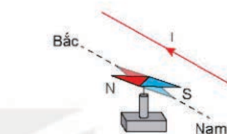
Hình 14.2. Thí nghiệm của Oersted (Ô-xét) về tương tác giữa dòng điện và kim nam châm
