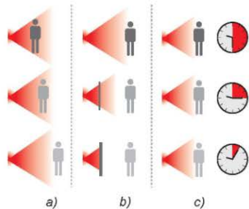
Hình 23.11. Ba nguyên tắc an toàn phóng xạ
