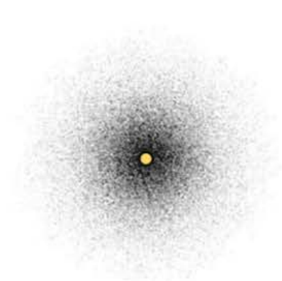
b) Mô hình đám mây electron
