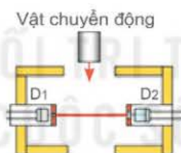
Hình 6.1. Cấu tạo cổng quang điện
