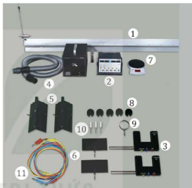
Hình 30.1. Bộ dụng cụ thí nghiệm xác định động lượng của hai vật trước và sau va chạm
