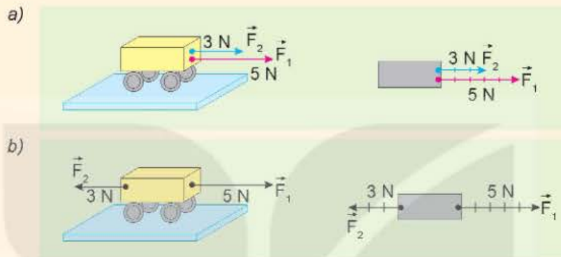
Hình 13.2. Tổng hợp hai lực cùng phương
