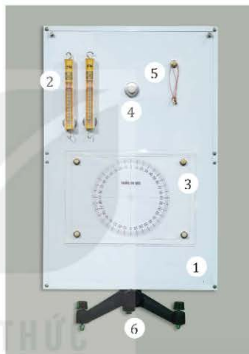
Hình 22.1. Bộ thí nghiệm tổng hợp hai lực đồng quy
