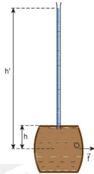
Hình 34.11 Thí nghiệm làm vỡ thùng gỗ tôn-nô của Pascal
